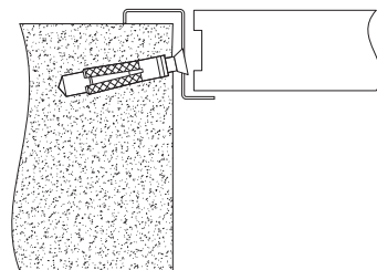
TELAIO A "Z" A TASSELLARE "Z" BOLT-IN FRAME
