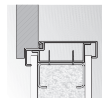
montajul tocului de colț 100 mm pe zid din gips-carton
