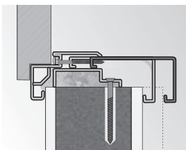
grosimea zidului interval de reglare
